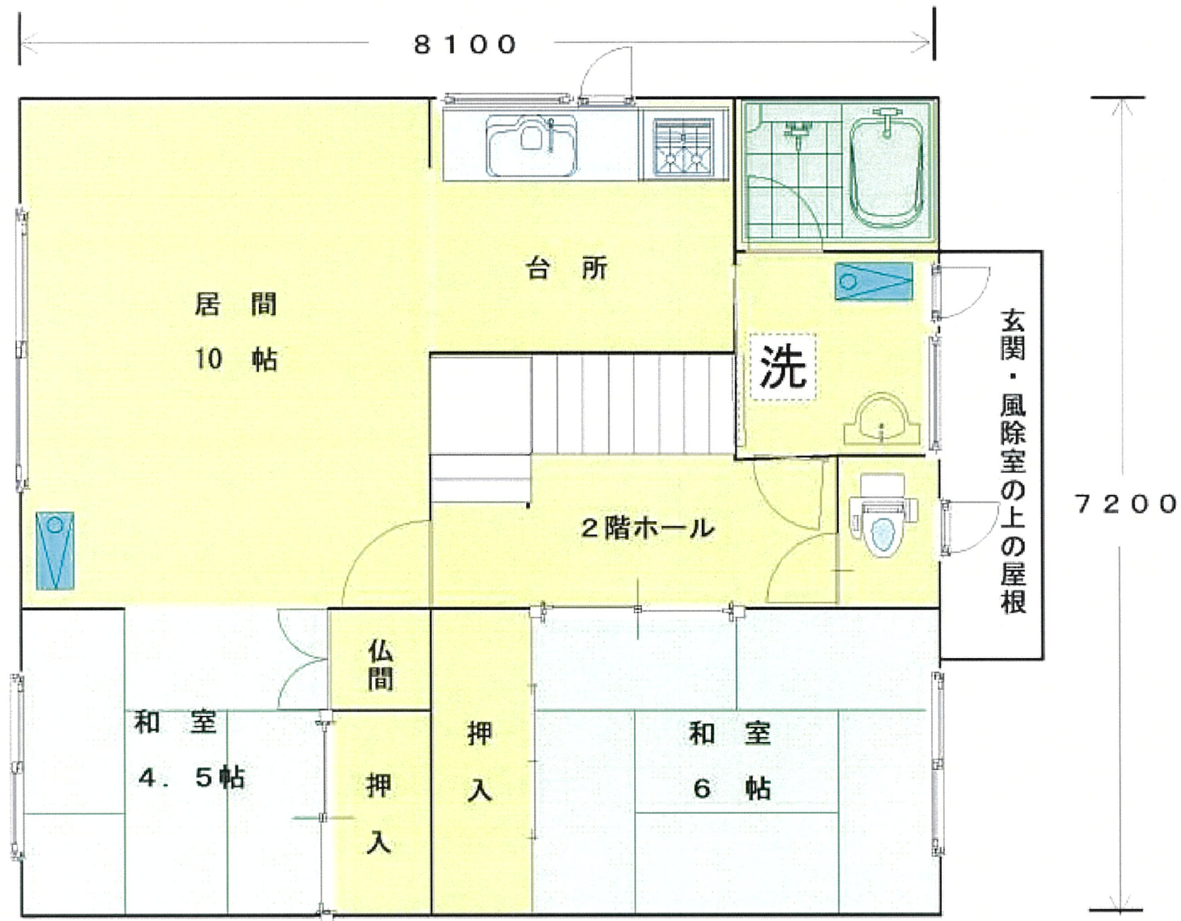
2階平面図 現況を優先します
